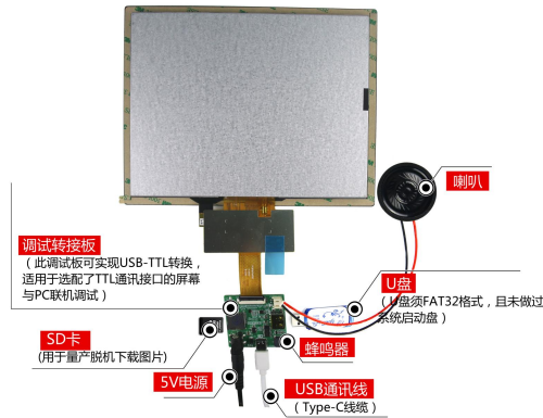
图 1-4 调试工具图
