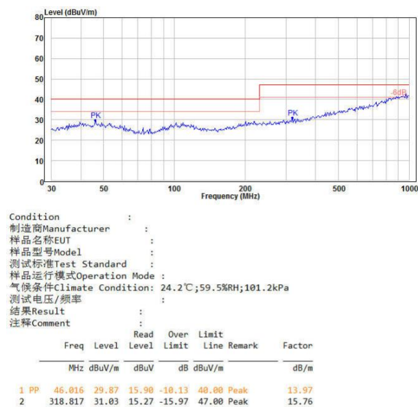
图 6-5 RE 测试水平方向
