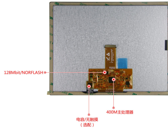
图 1-3 硬件配置图
