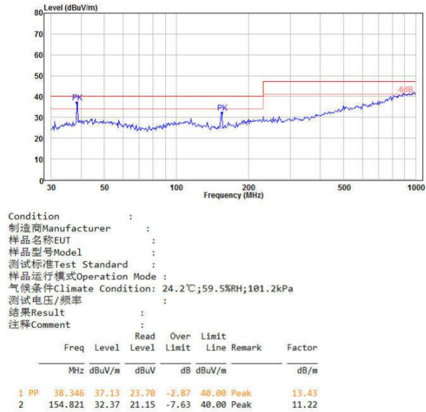
图 6-6 RE 测试垂直方向
